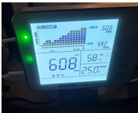
Bild: CO 2 -Messung, Luftfeuchte und Temp.
