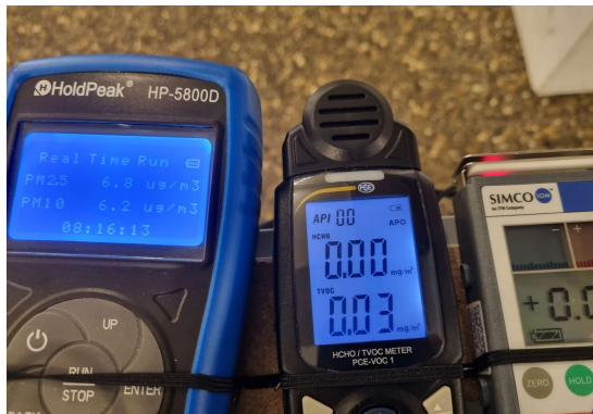
Bild: Messaufbau
