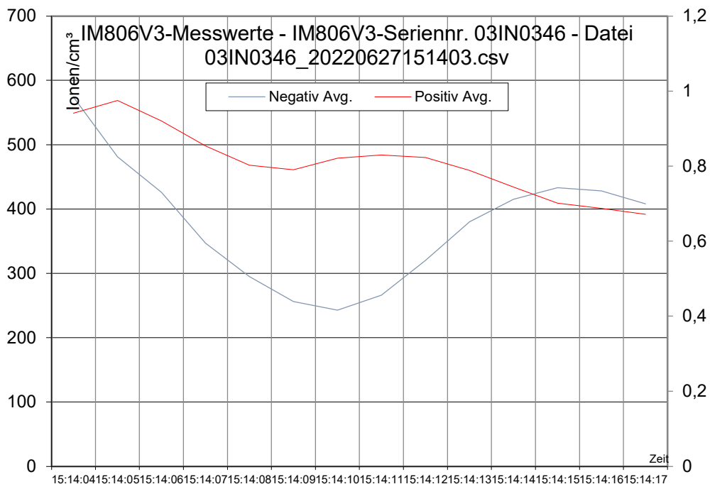
Diagramm: Luftwerte vor Schulgebäude
