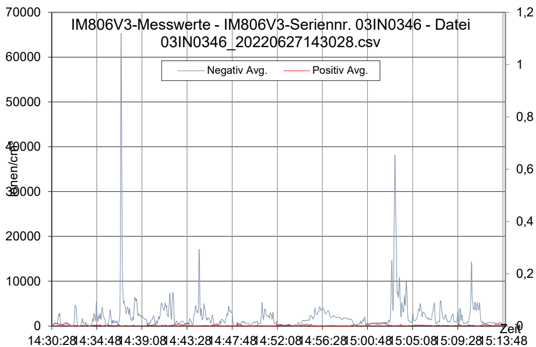
Diagramm: Luftwerte Ionisation in Klassenzimmern; Die Senken sind Bewegungen im Flur oder Pause auf Hof
