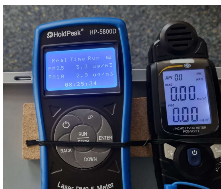
Bild: Feinstaubmessgerät HOLDPEAK® re. PCE-HCHO und TVOC-Messgerät
